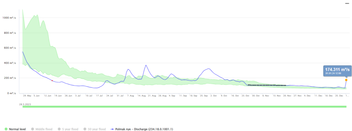
Figur 2: Figuren viser vannføringen ( \text{m}^3/\text{s} ) målt ved NVEs målestasjonen i Polmak fra mai til januar. Heltrukken linje viser vannføringen i 2023. Det grønne feltet viser 25 til 75 persentilene, som sammenligner dagens registrering med vannføringen på samme dato fra mange tidligere år.
